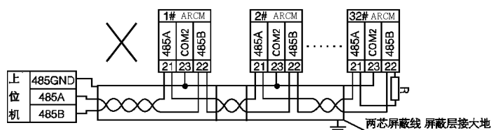
错误接线方式：通讯电缆屏蔽层接485GND
