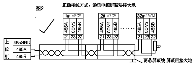
正确接线方式：通讯电缆屏蔽层接公共地但不允许同时接大地
