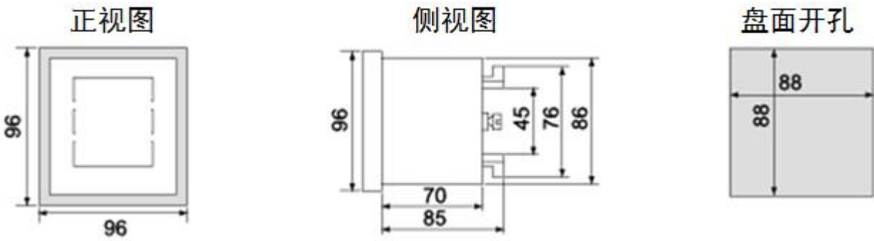
ACR220ELH 尺寸
