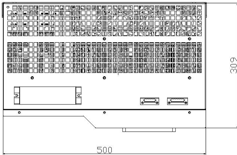
图 2-14 ANSVG-100kvar 壁挂模块机箱俯视图
