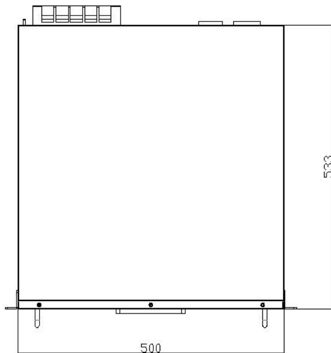
图 2-11 ANSVG-100kvar 模块机箱俯视图
