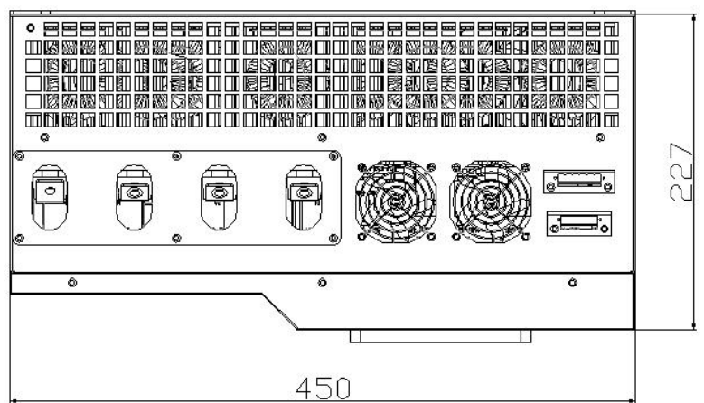
图 2-8 ANSVG-50kvar、ANSVG-75kvar 壁挂模块机箱俯视图
