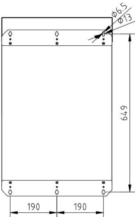
图 2-7 ANSVG-50kvar、ANSVG-75kvar 壁挂模块机箱后视图
