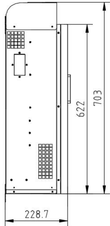
图 2-6 ANSVG-50kvar、ANSVG-75kvar 壁挂模块机箱侧视图
