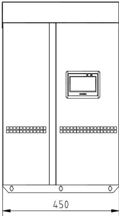
图 2-5 ANSVG-50kvar、ANSVG-75kvar 壁挂模块机箱主视图
