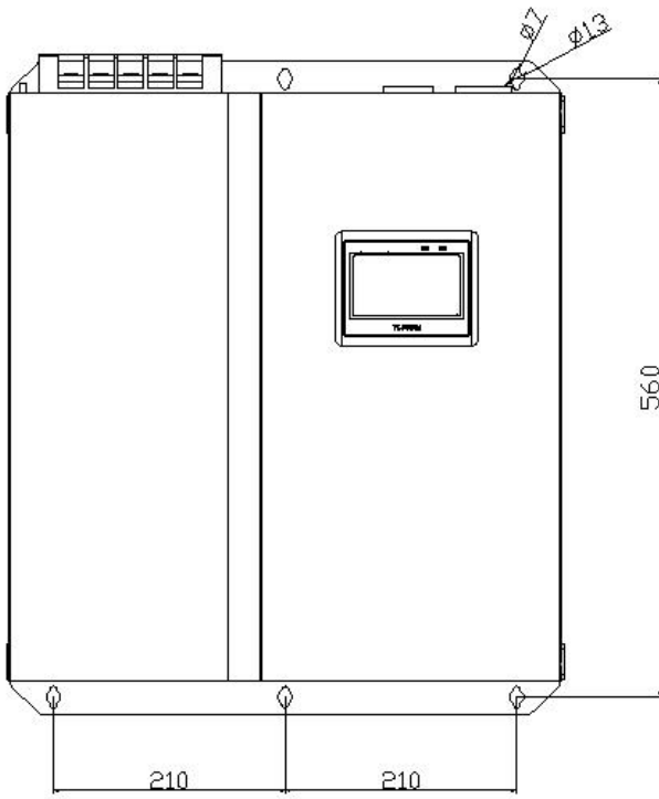
图 2-12 ANSVG-100kvar 壁挂模块机箱主视图
