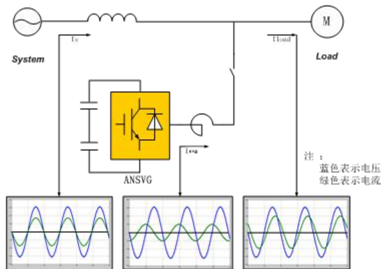
图2-19 ANSVG 原理图
