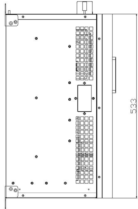
图 2-13 ANSVG-100kvar 壁挂模块机箱侧视图
