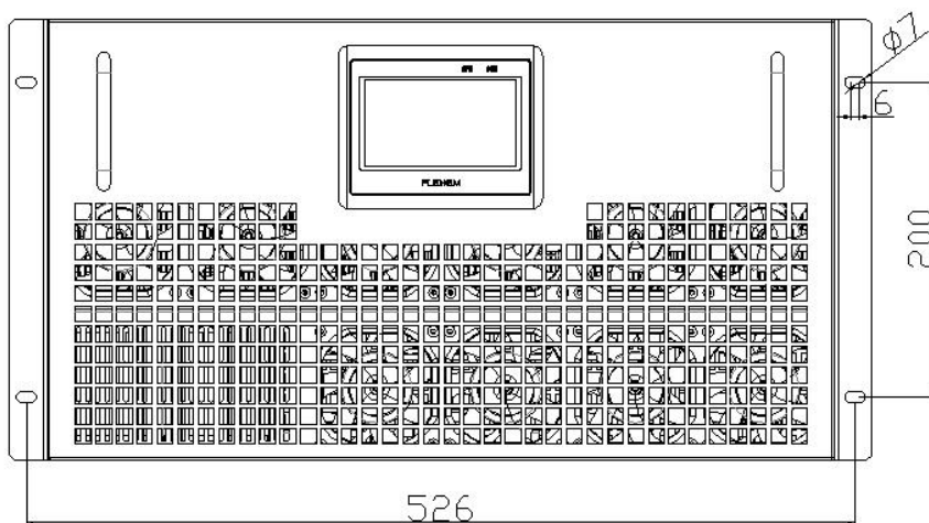
图 2-9 ANSVG-100kvar 模块机箱主视图
