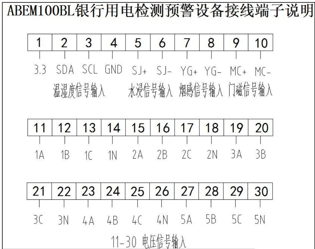
图 5 接线端子定义
