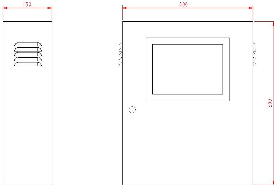
图3 设备外形尺寸图
