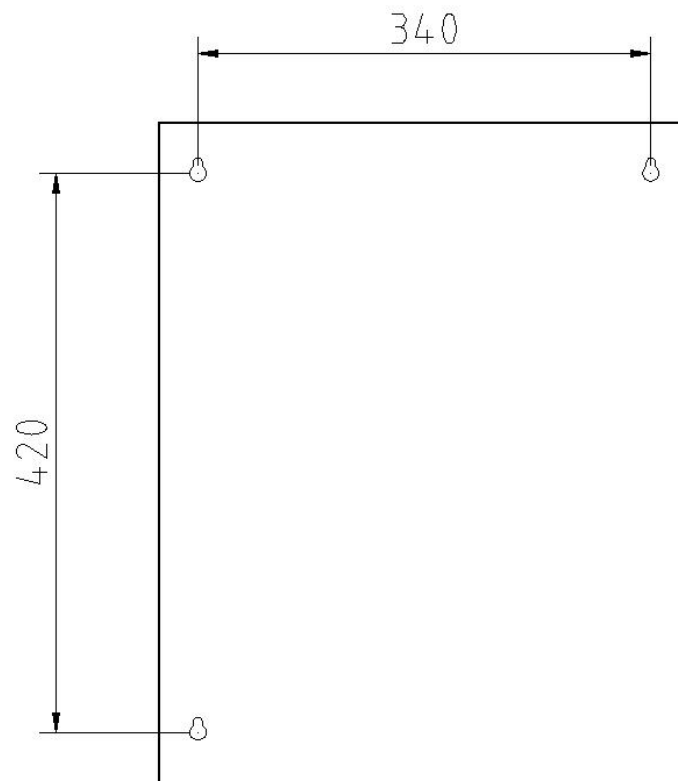
图4 设备安装尺寸图
