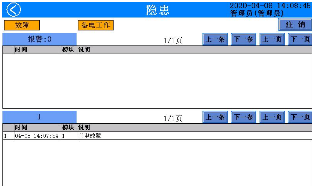
图 10 隐患页面
