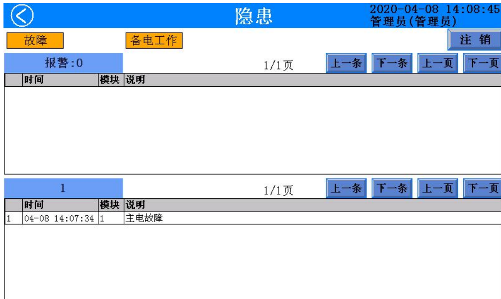
图 8 系统主界面
