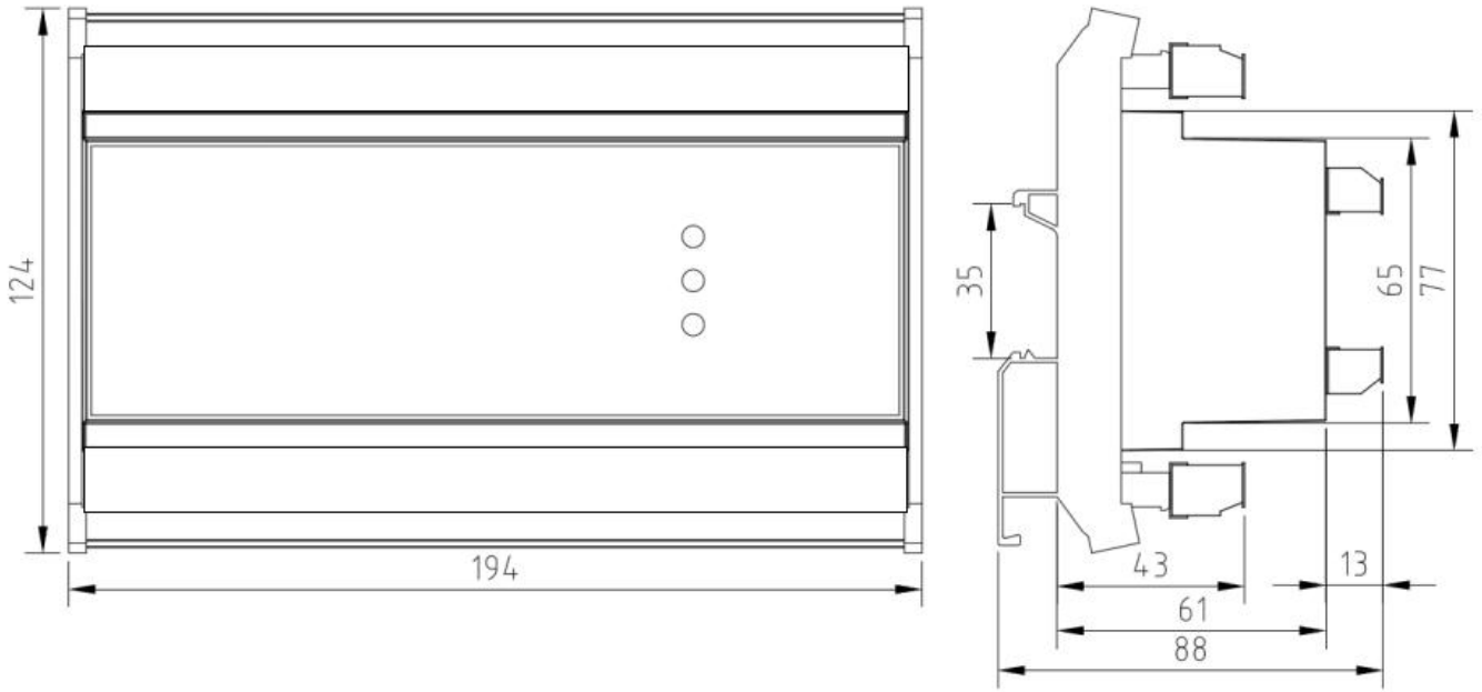
单表尺寸图
