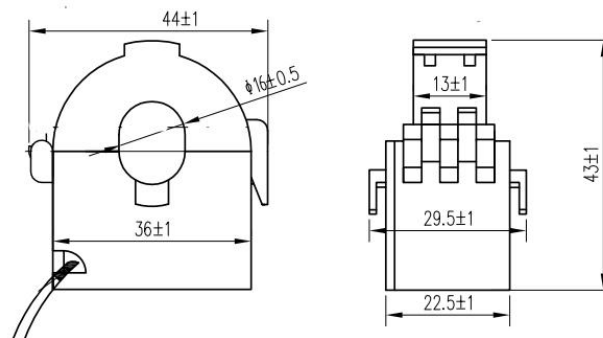
外置互感器外形尺寸
