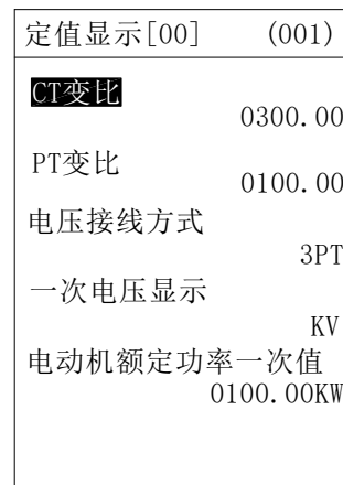
图 3.12 定值显示
