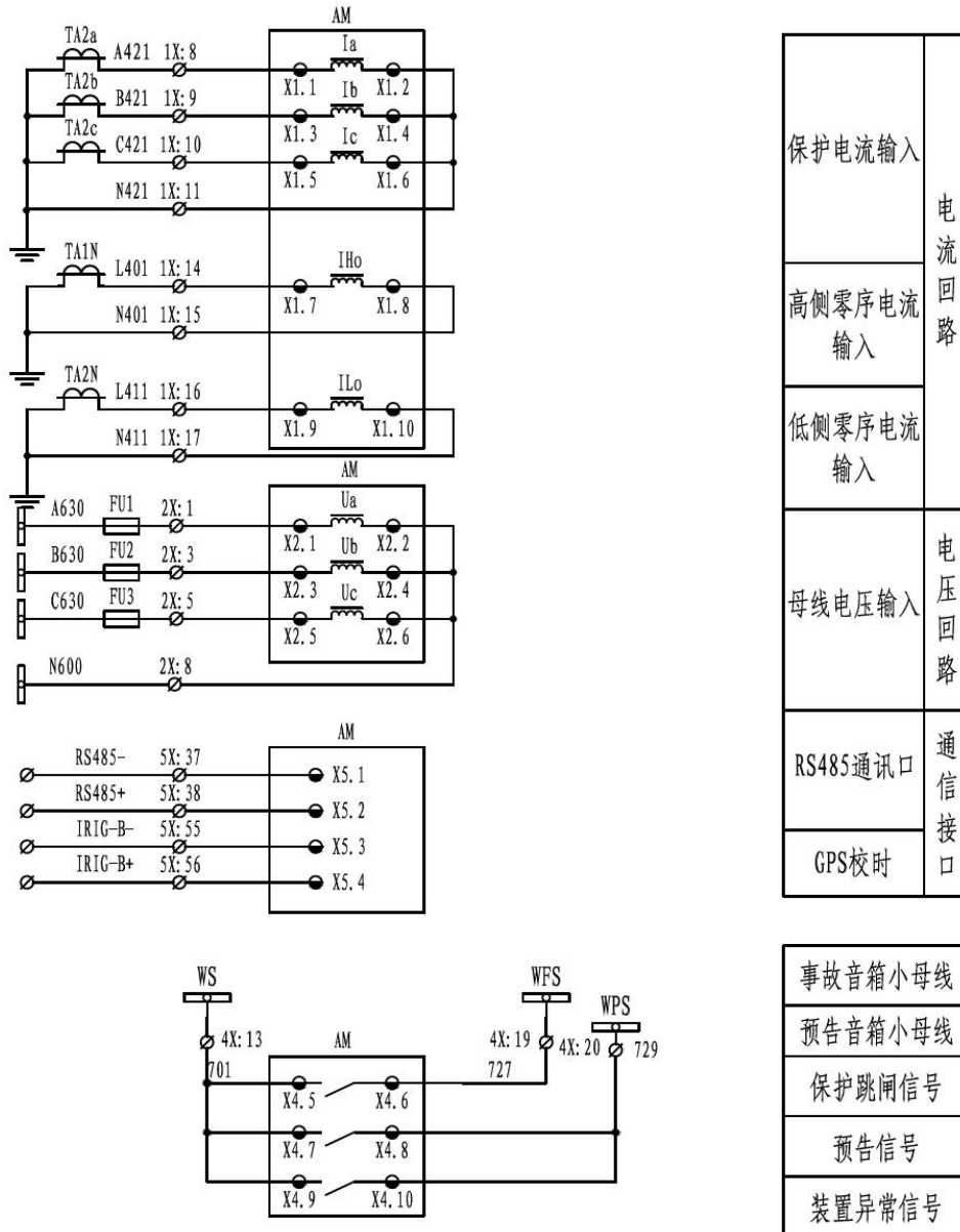
图 1.24 AM3SE-I 二次原理图 (三)
