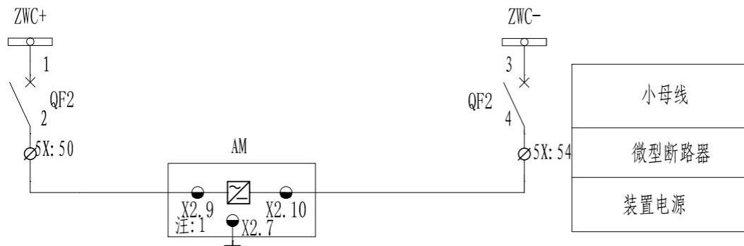
图 1.22 AM3SE-I 二次原理图 (一)
