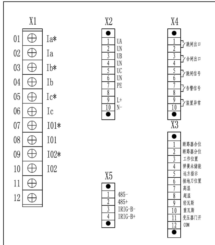
图 1.20 AM3SE-I 电气接线图
