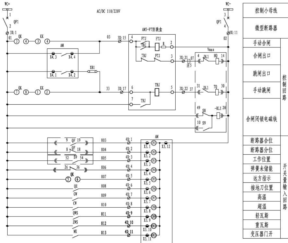
图 1.23 AM3SE-I 二次原理图 (二)
