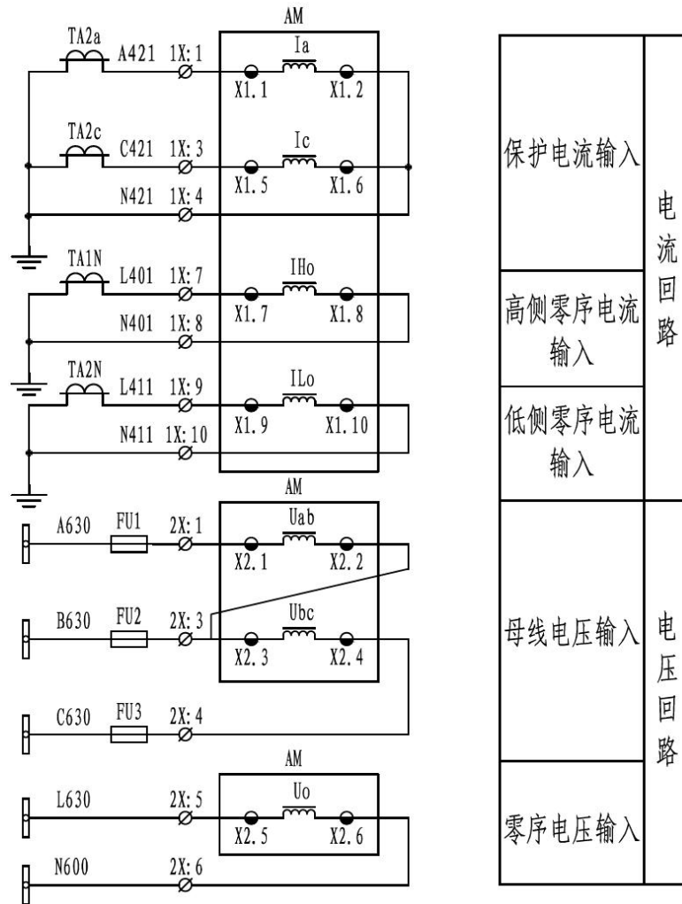
图 1.21 2PT 2CT 接线方法
