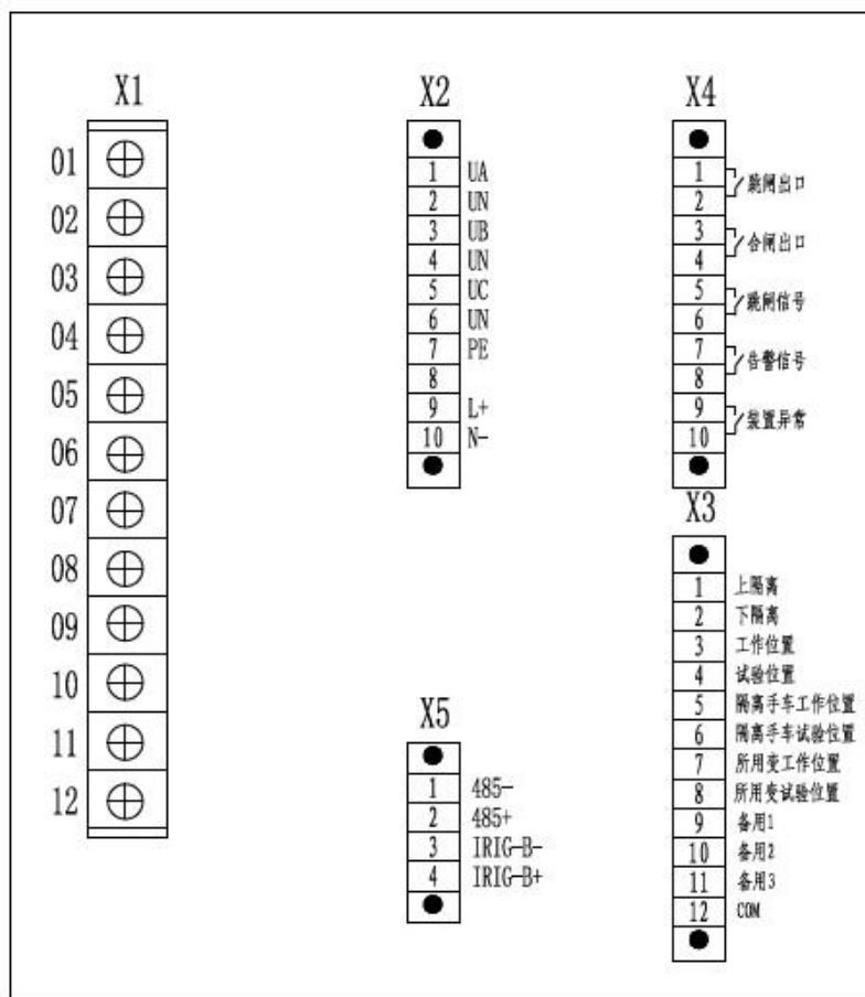
图 2.5 AM3SE-U 电气接线图
