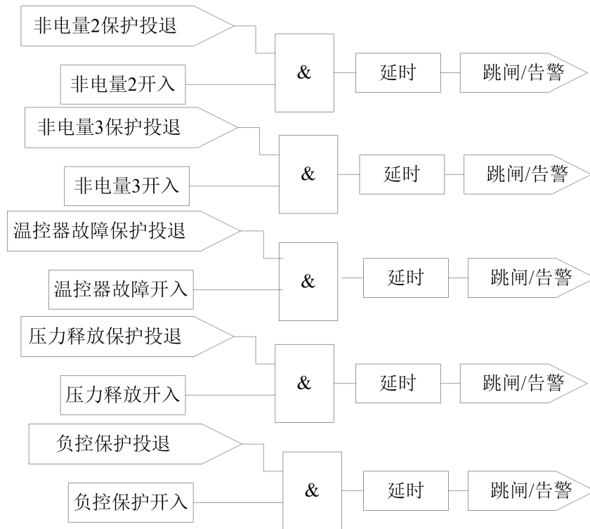
图 2.13 非电量保护逻辑
