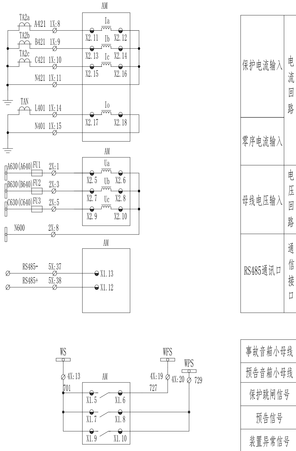
图 2.21 AM2SE 二次原理图（三）
