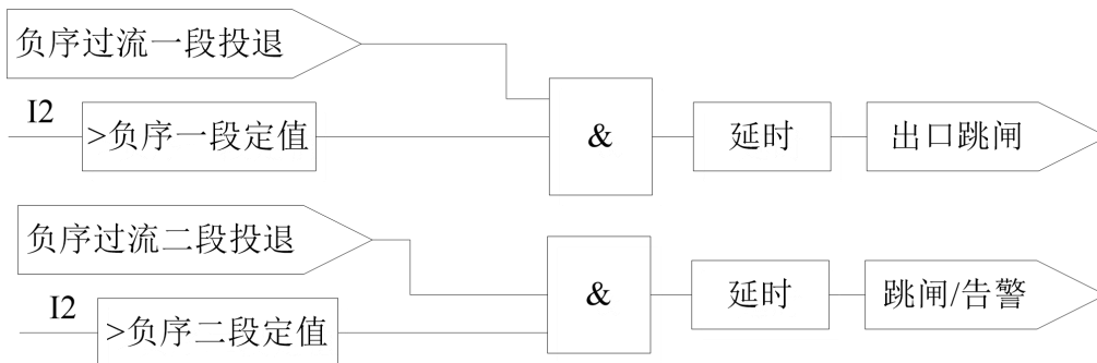
图 2.11 两段式负序过流保护逻辑
