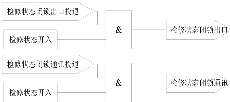
图 2.16 检修状态闭锁逻辑
