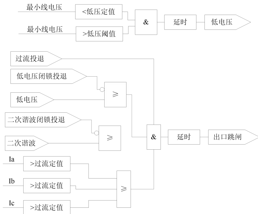
图 2.1 三段式过流保护逻辑
