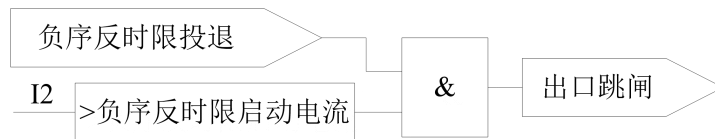
图 2.12 负序反时限过流保护逻辑
