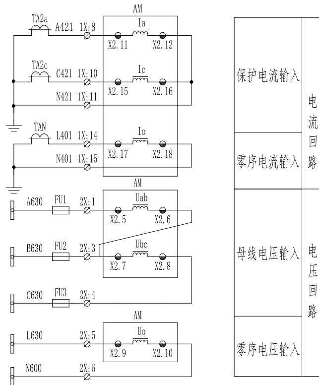
图 2.18 2PT 2CT 接线方法
