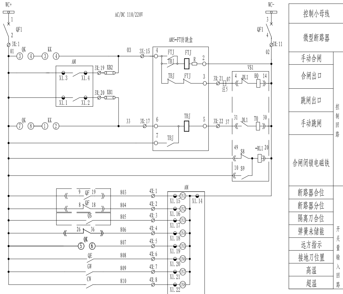
图 2.20 AM2SE 二次原理图 (二)
