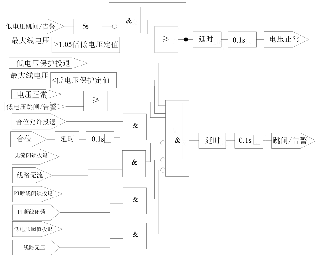
图 2.10 低电压保护逻辑
