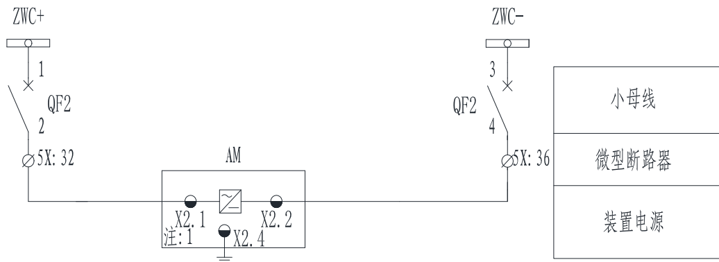
图 2.19 AM2SE 二次原理图 (一)
