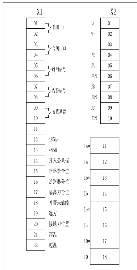
图 2. 17 AM2SE-V 电气接线图（-H 和 -V 背后端子定义完全相同）
