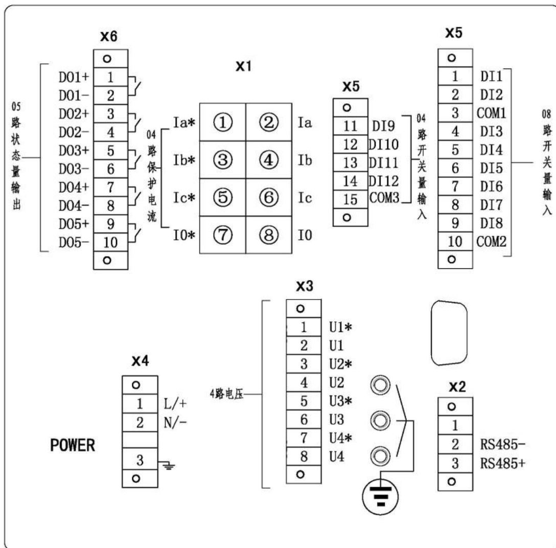
图 5.1 AM4 电气接线图
