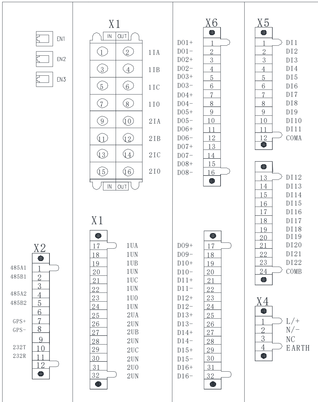
图 3.3 背部端子图
