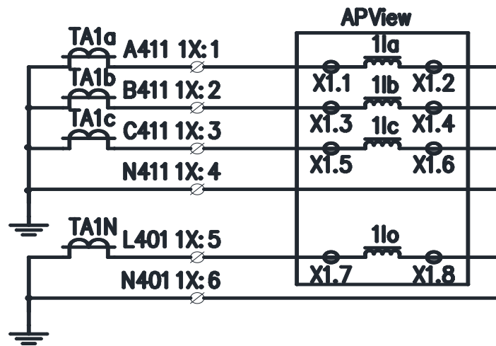
图 3.5 3CT 电流接线
