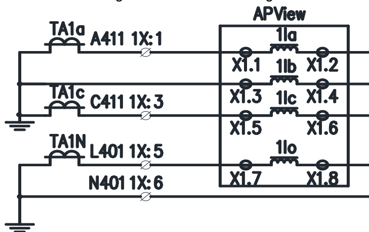
图 3.6 2CT 电流接线
