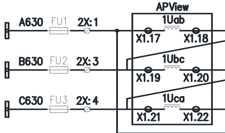
图 3.8 2PT 电压接线 Fig. 3.8 2PT Voltage wiring
