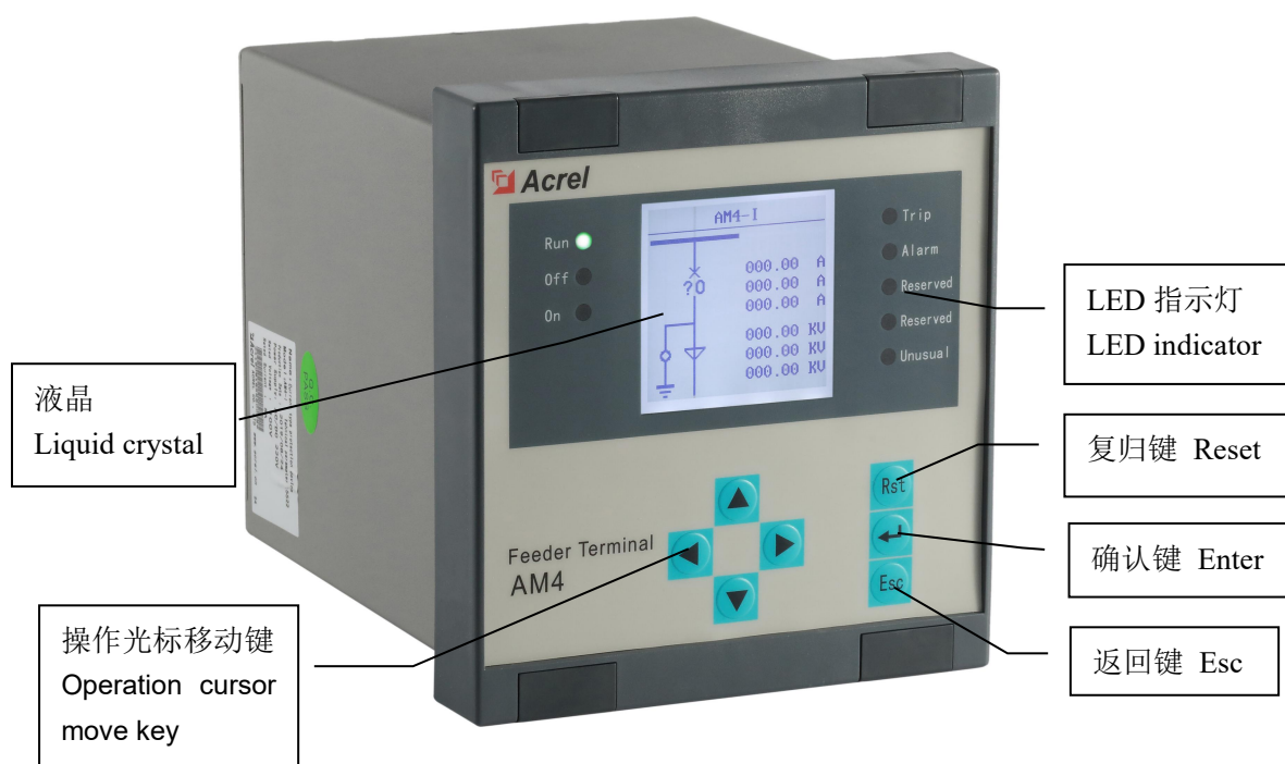
图 3.1 AM4 前面板
