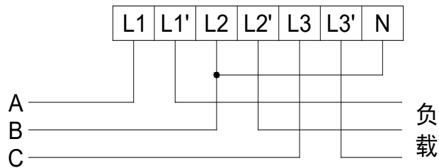
DTSY1352 三相三线直接接入
