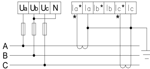
DTSY1352 三相三线经互感器接入
