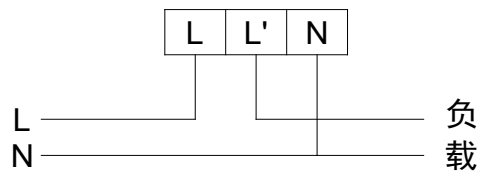
DDSY1352 接线图
