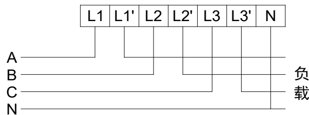
DTSY1352 三相四线直接接入
