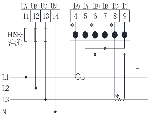
3P4L/2CT (仪表设置为BP4L) 注②
