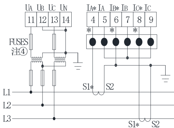
3P3L/2PT+2CT-2 (仪表设置为BP3L) 注③
